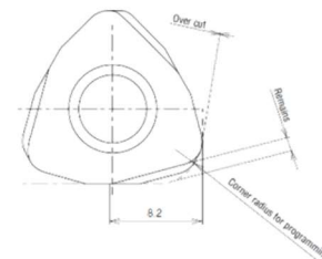
Theoretischer Eckenradius
